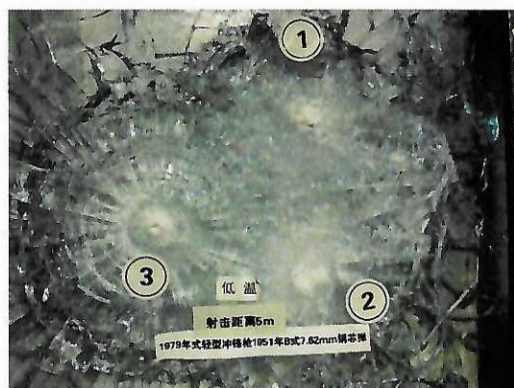
图五: 低温条件下, 防弹复合玻璃中弹后, 正面弹伤状态
