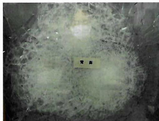
图二: 常温条件下, 防弹复合玻璃中弹后, 背面弹伤状态
